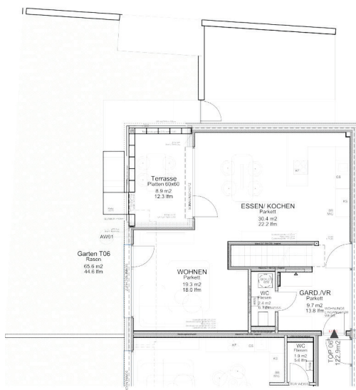
HAUS B: TOP 06 OBERGESCHOSS
